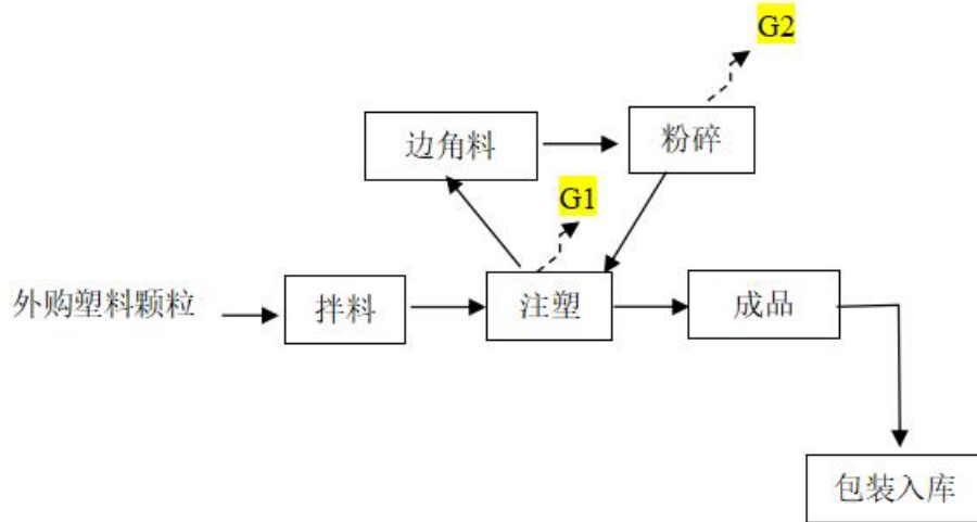
图 3-3 项目工艺流程图
