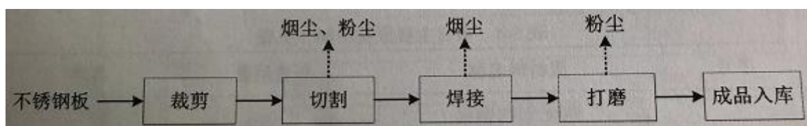
图 3-5 料桶工艺流程图
