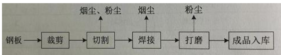
图 3-3 卷管工艺流程图
