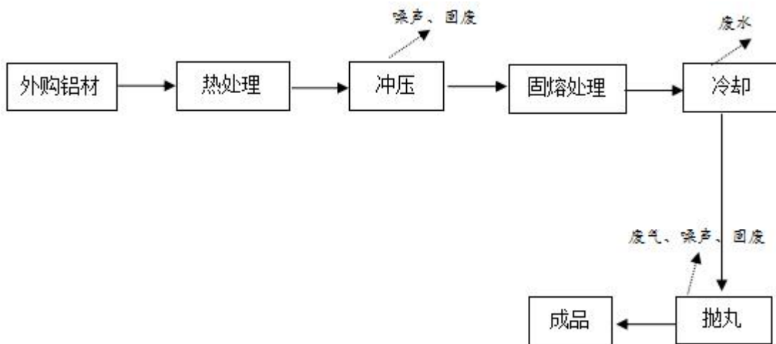
图 3-3 工艺流程图
