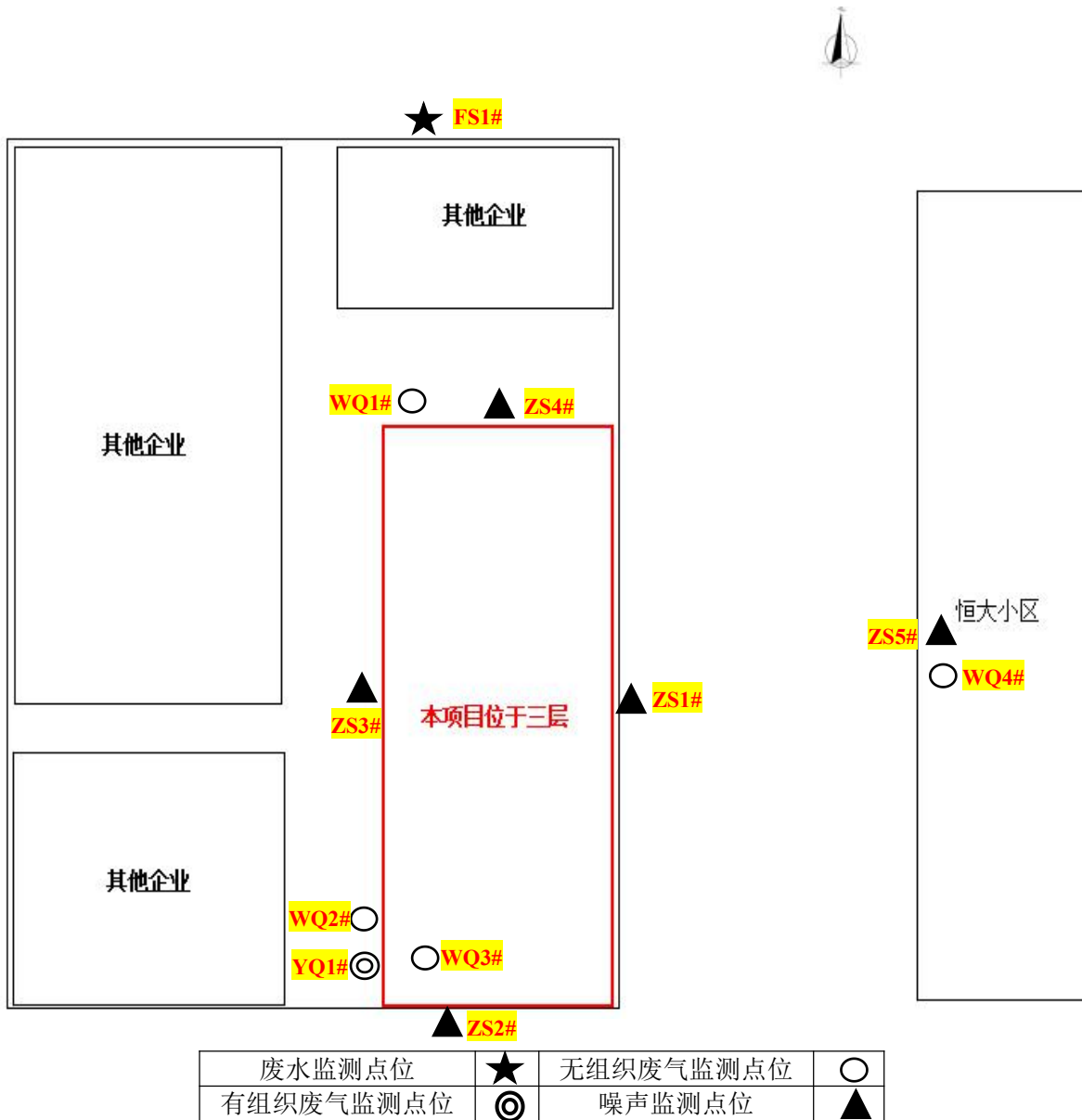
图 7-1 项目监测点位示意图
