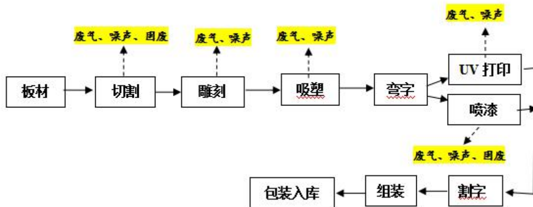
图 3-3 项目工艺流程图
