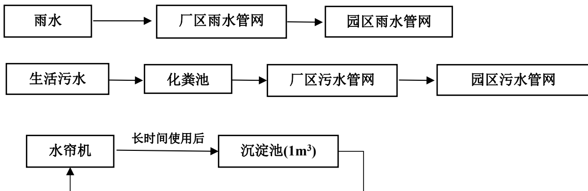
图 4-1 项目废水防治措施
