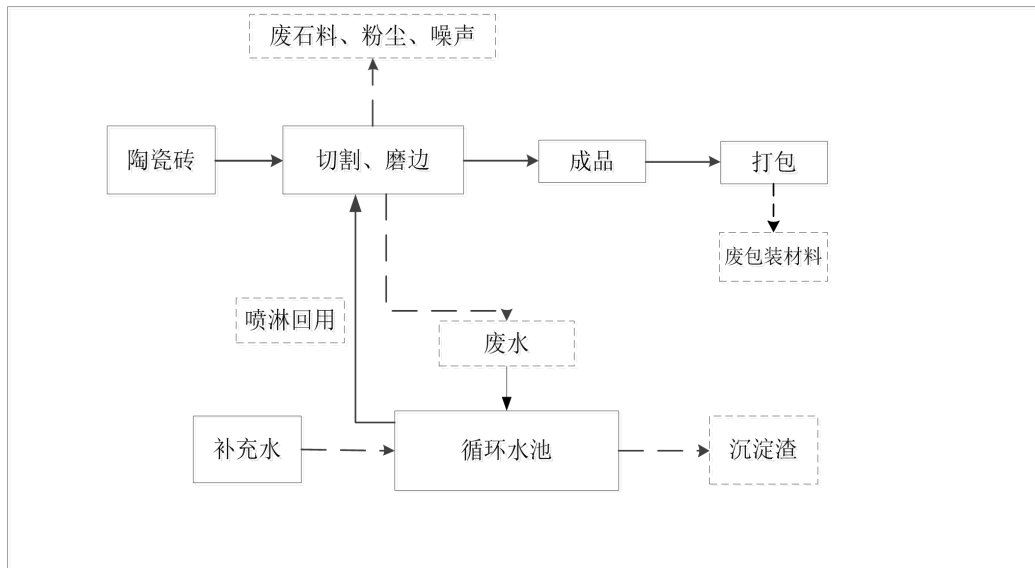
图 3-3 项目工艺流程图
