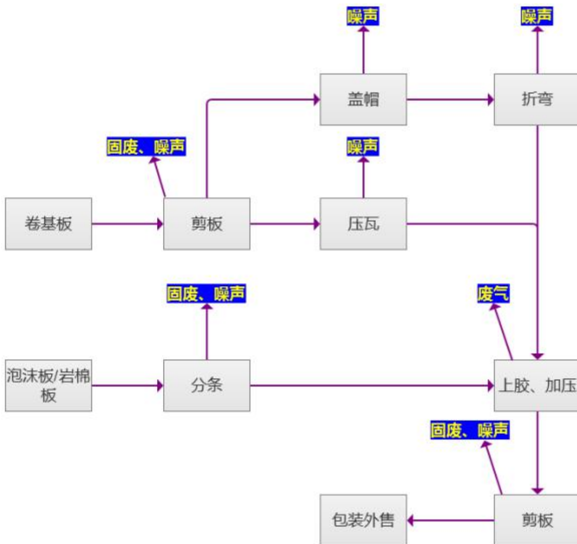
图 3-3 项目工艺流程图
